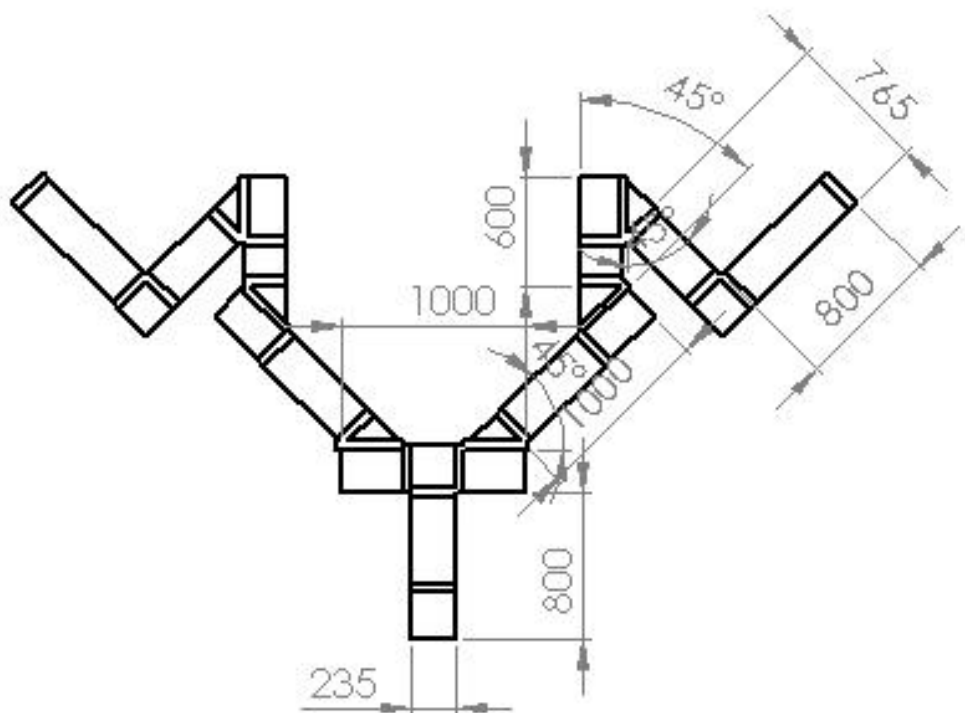
圖四「歹路不可行」場地尺寸圖
